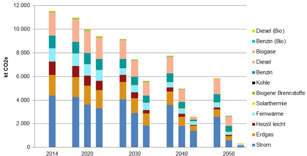
Abbildung 3: Treibhausgas-Emissionen nach Energieträgern in 2050 in allen Szenarien. Linke Säule: Referenzszenario, Mitte: Szenario Klimaschutz moderat, rechts: Szenario Klimaneutrales München.
